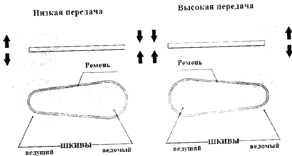
Принцип работы клиноременного вариатора
